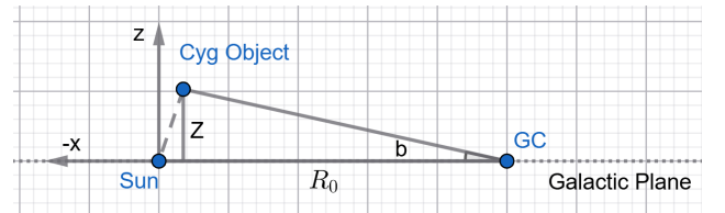
FIGURE 2 – Géométrie de projection selon l'axe vertical ( Z ).
