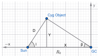
FIGURE 1 – Géométrie de projection dans le plan galactique ( X, Y ).
